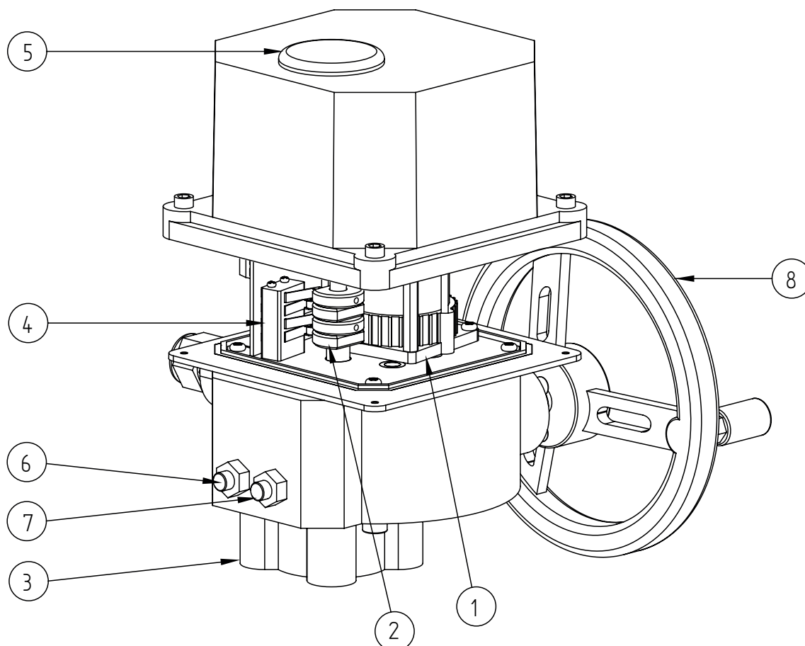
Servomoteur UMC 15
