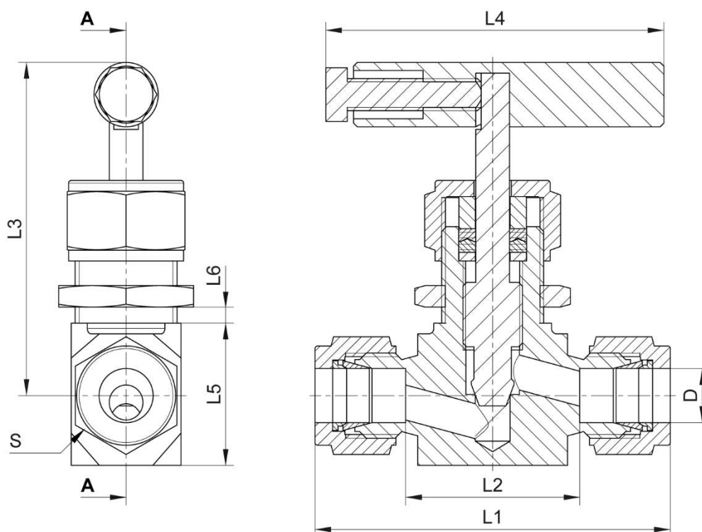
COUPE A-A
