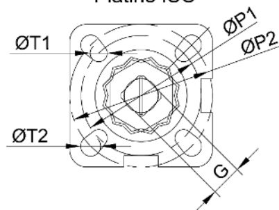
Platine ISO
