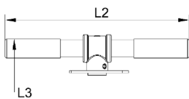
Poignée DN80 - 200 (3" - 8")
