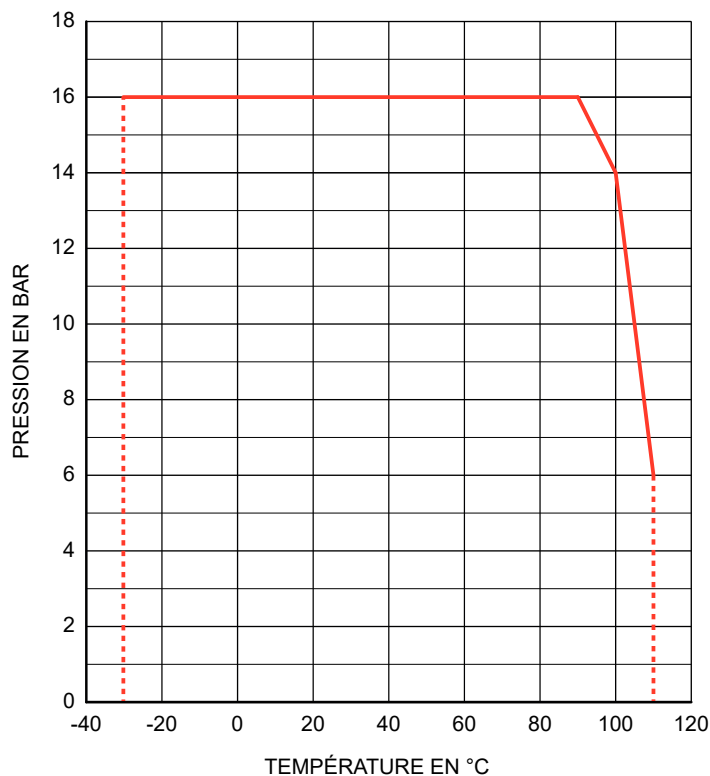
58429 : Manchette EPDM
