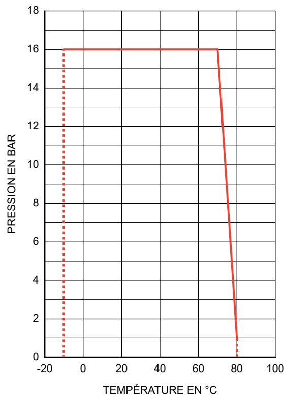
58422 : Manchette NBR
