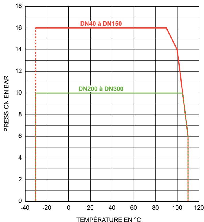
58459 : Manchette EPDM
