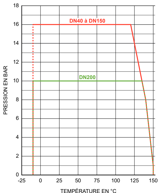
58453 : Manchette FKM
