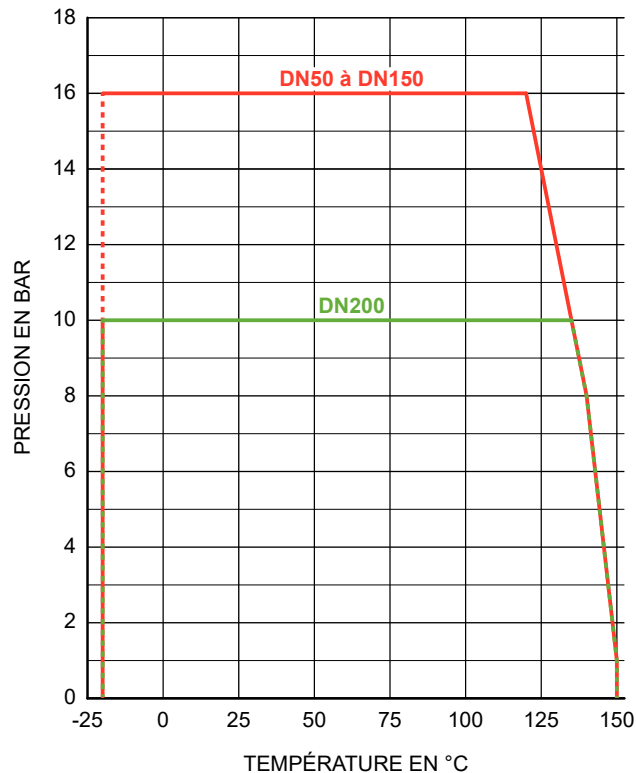
58454 : Manchette Silicone
