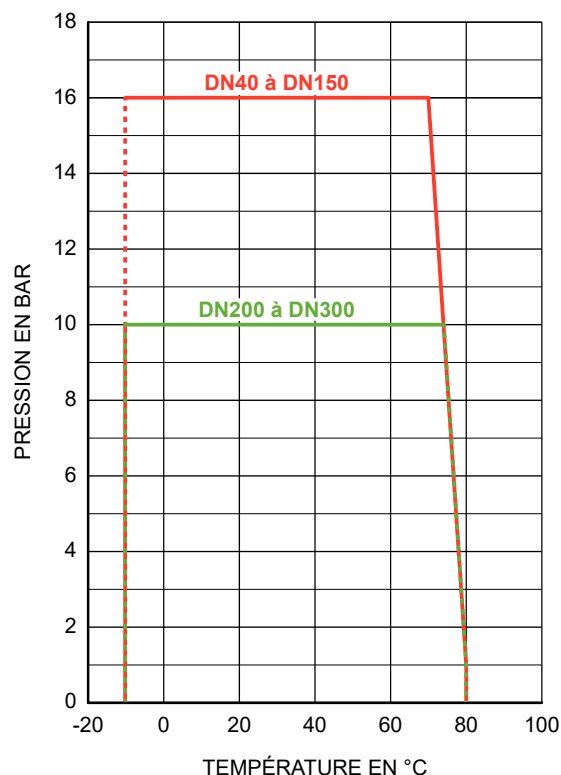
58452 : Manchette NBR
