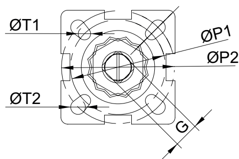
Platine ISO
