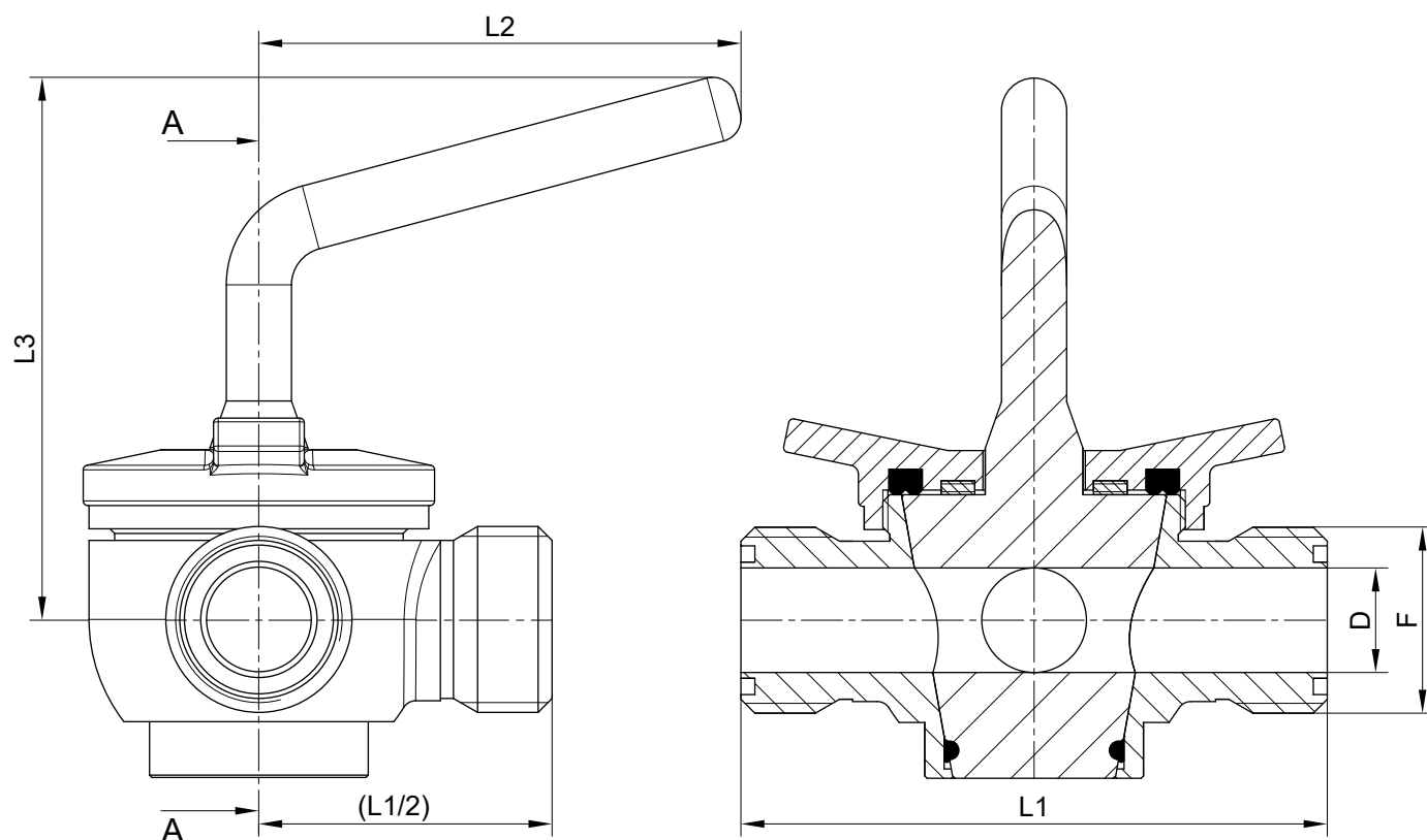
COUPE A-A
