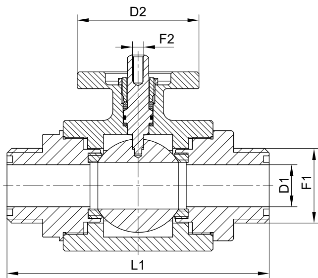
COUPE A-A
