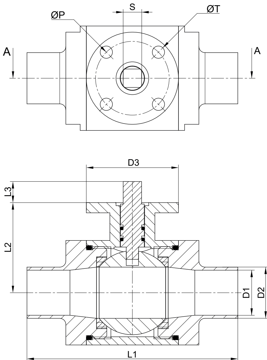
COUPE A-A
