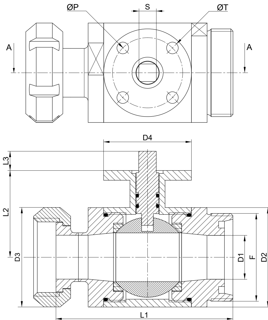
COUPE A-A
