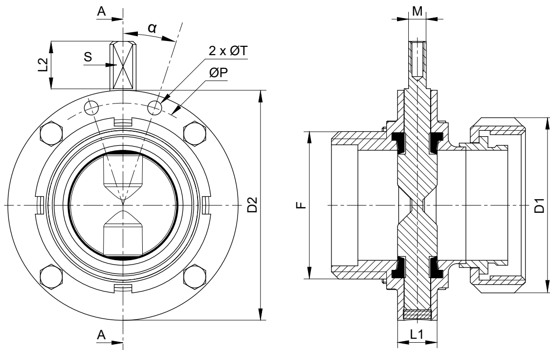
COUPE A-A
