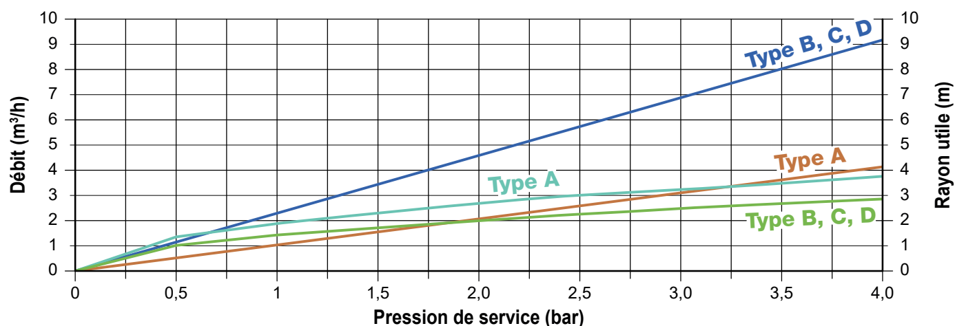
Relation pression, débit et rayon utile pour boule catégorie BL17
