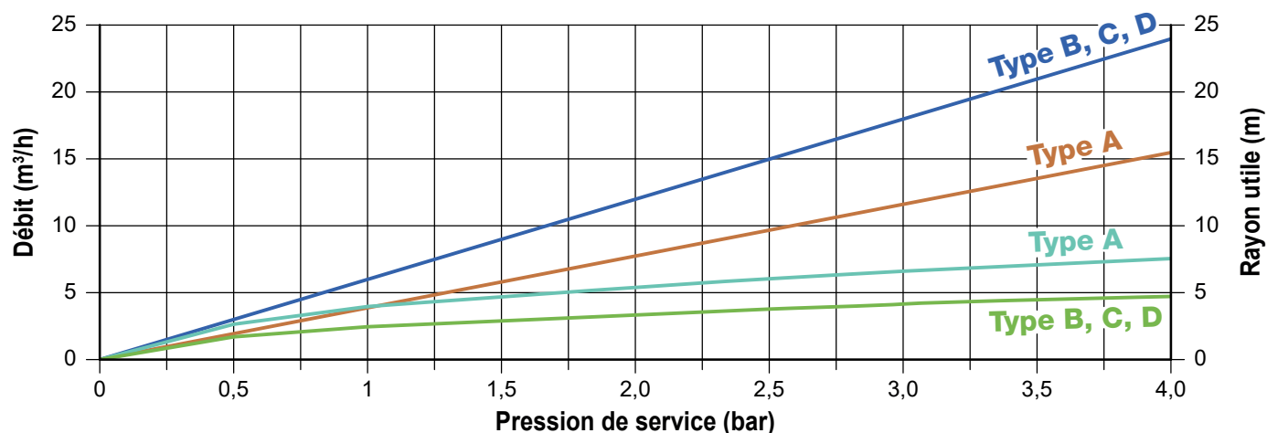
Relation pression, débit et rayon utile pour boule catégorie BL15
