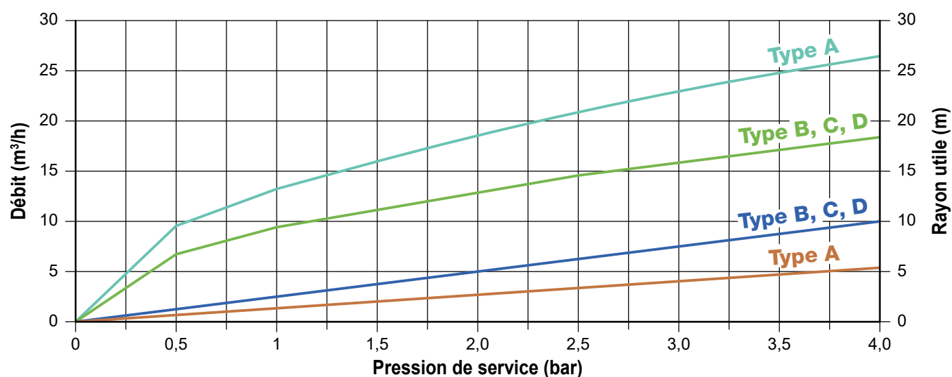
Relation pression, débit et rayon utile pour boule catégorie BL3
